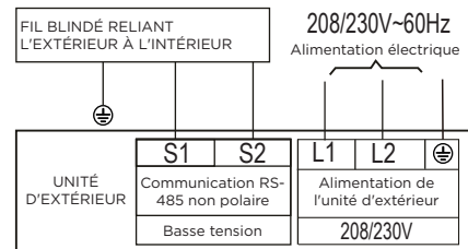
Unité extérieure A
