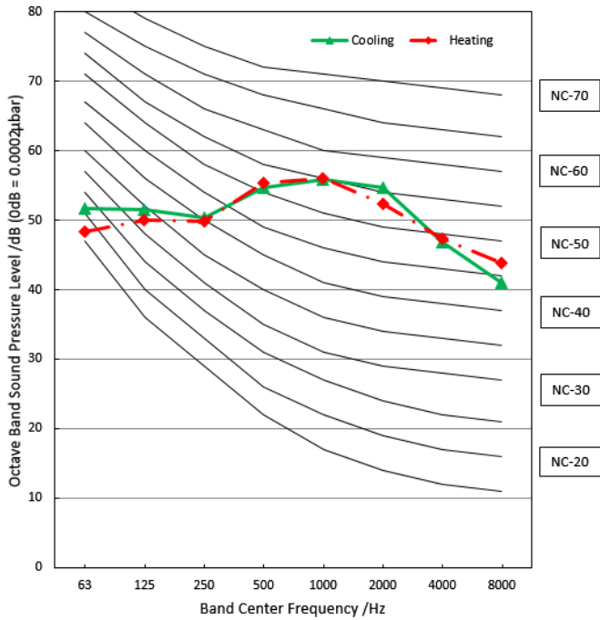
MOE30U-48HFN1-MR0
