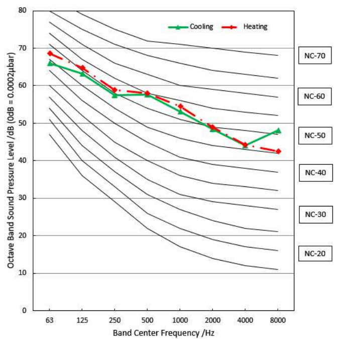
MOE31U-36HFN1-M
