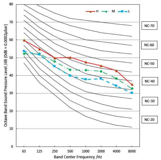
MVC-60HWFN1-M
