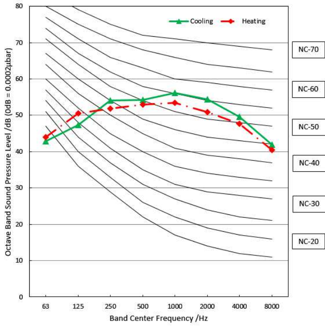
MOE30U-48HFN1-MR0
