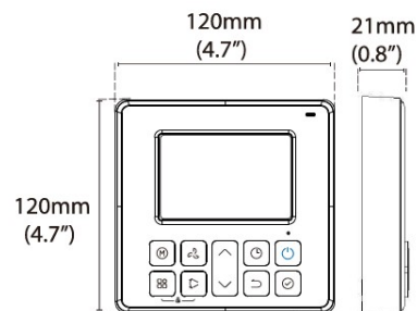
Drawing dimensions are nominal. / Les dimensions du dessin sont nominales.
