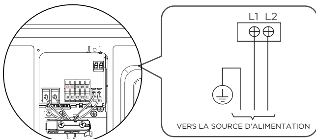
Unité extérieure A
